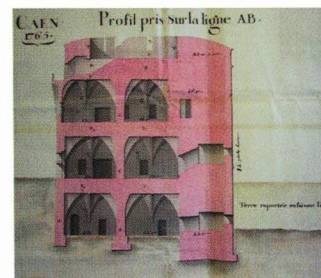
Coupe de la tour Châtimoine, 1765, SHD Vincennes
